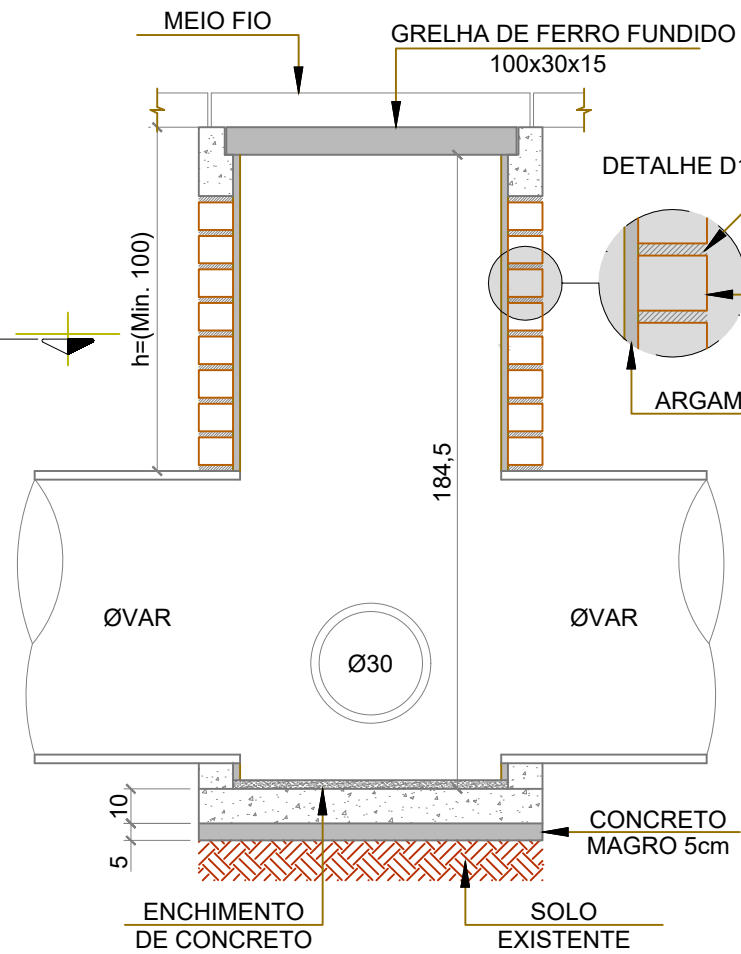
CORTE A-A
