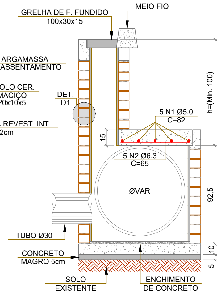
CORTE B-B
