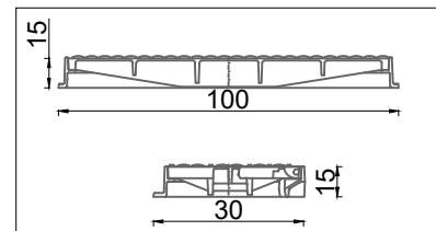
DETALHE GRELHA DE F. FUNDIDO
