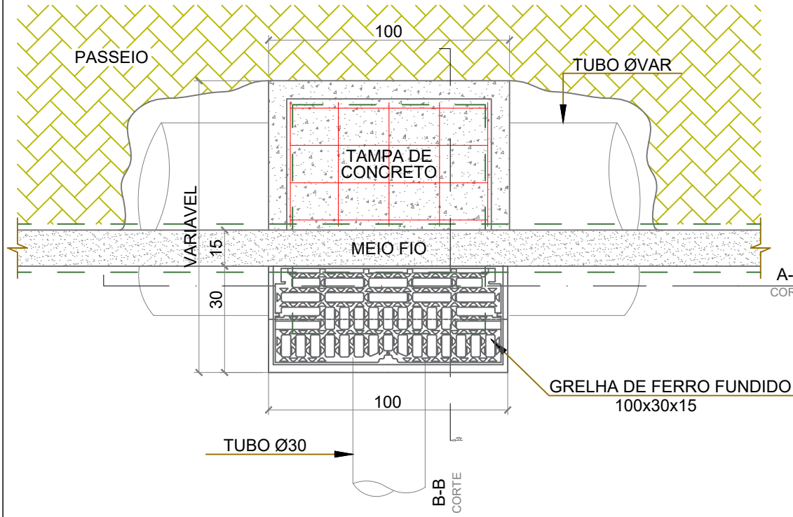
DETALHE GRELHA DE F. FUNDIDO
