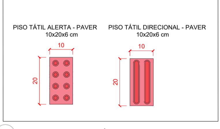
3 DETALHE - PISO TÁTIL DE ALERTA E DIRECIONAL SEM ESCALA
