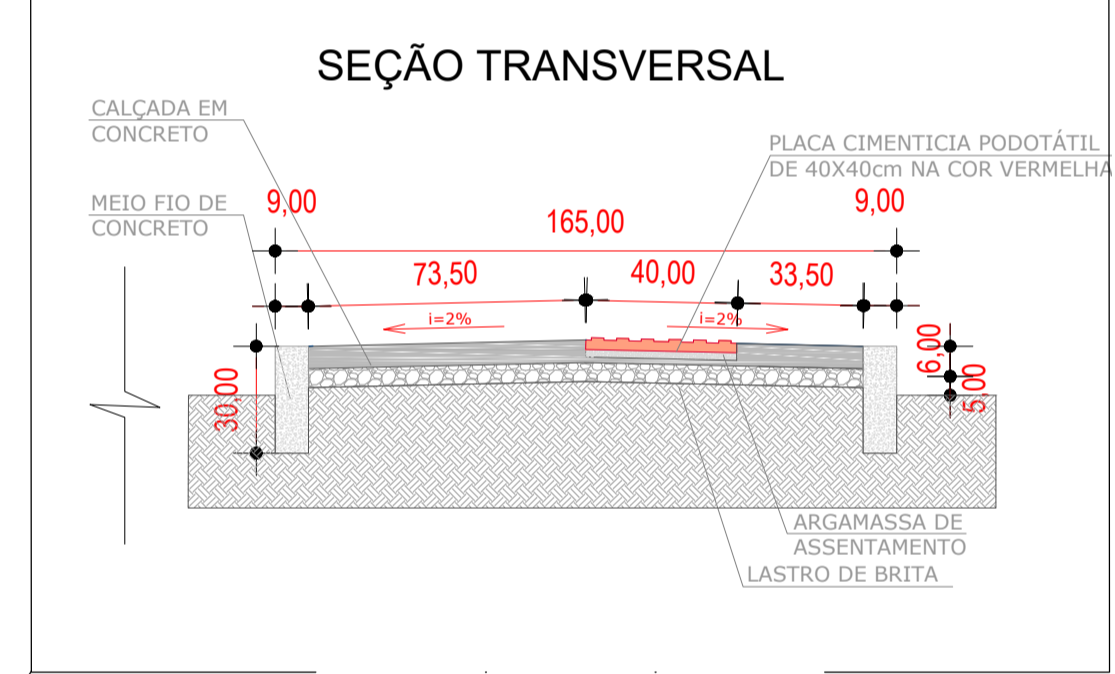
5 DETALHE - SEÇÃO TRANSVERSAL CALÇADA EM CONCRETO ESCALA 1:25
