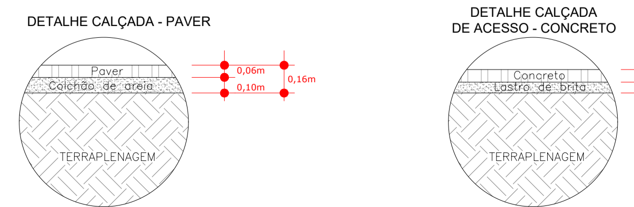
9 DETALHE - CALÇADAS SEM ESCALA
