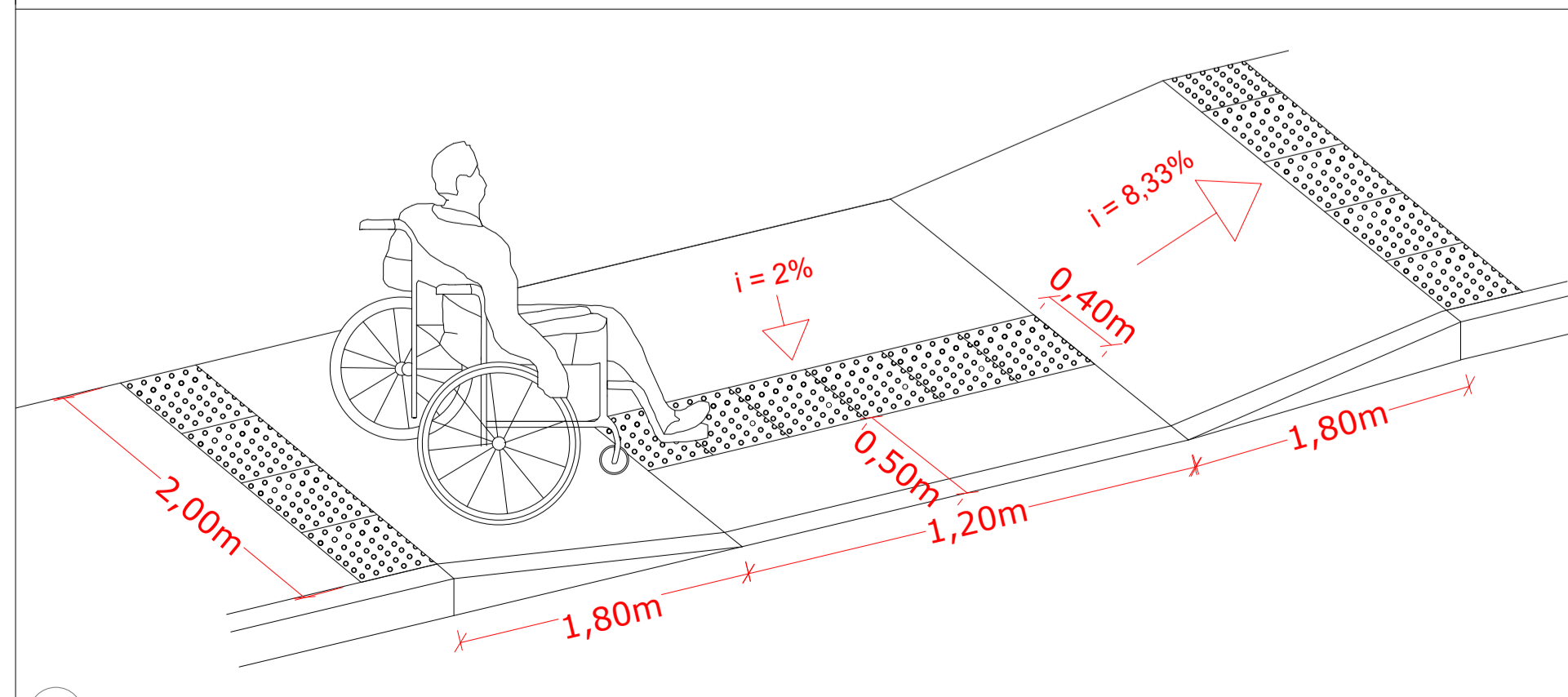
6 DETALHE - RAMPA DA CALÇADA EM PAVER SEM ESCALA
