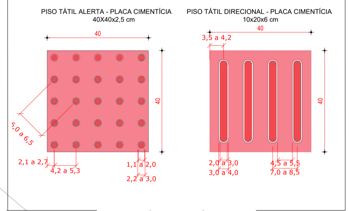
4 DETALHE - PISO TÁTIL DE ALERTA E DIRECIONAL SEM ESCALA
