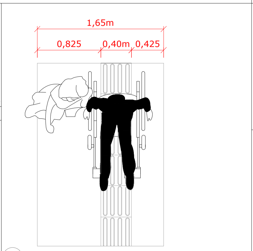
7 DETALHE - RAMPA DA CALÇADA EM CONCRETO SEM ESCALA
