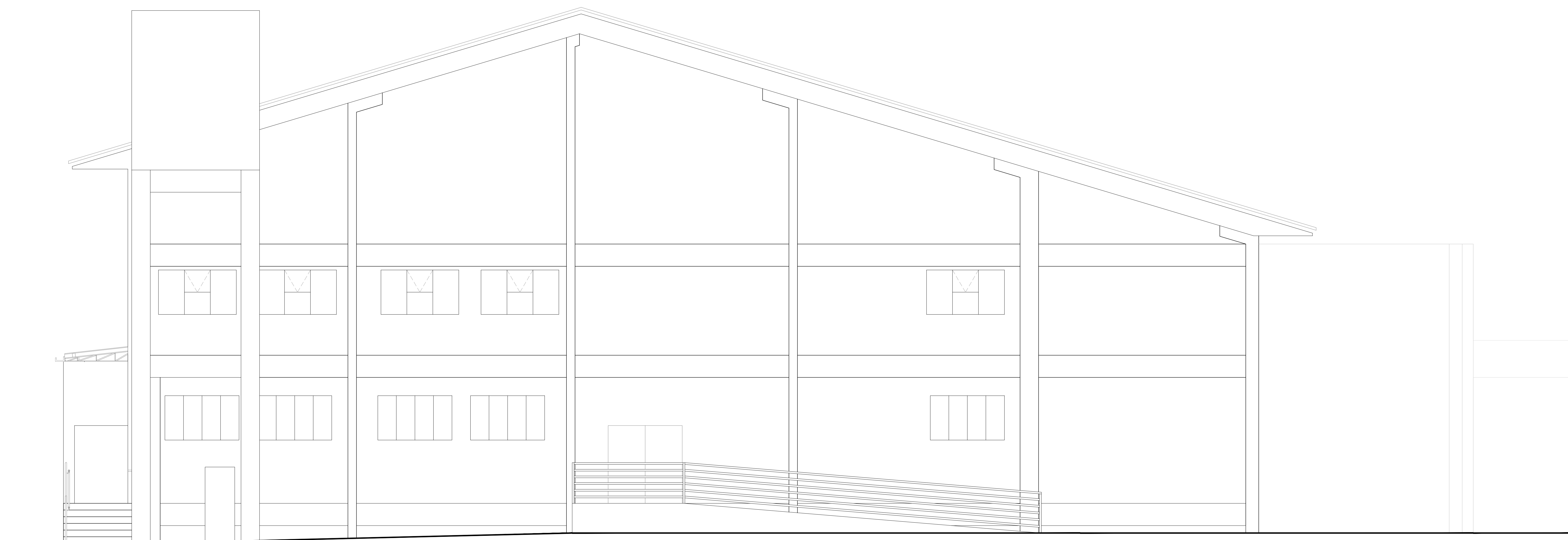
2 VISTA 02 ESCALA 1:50
