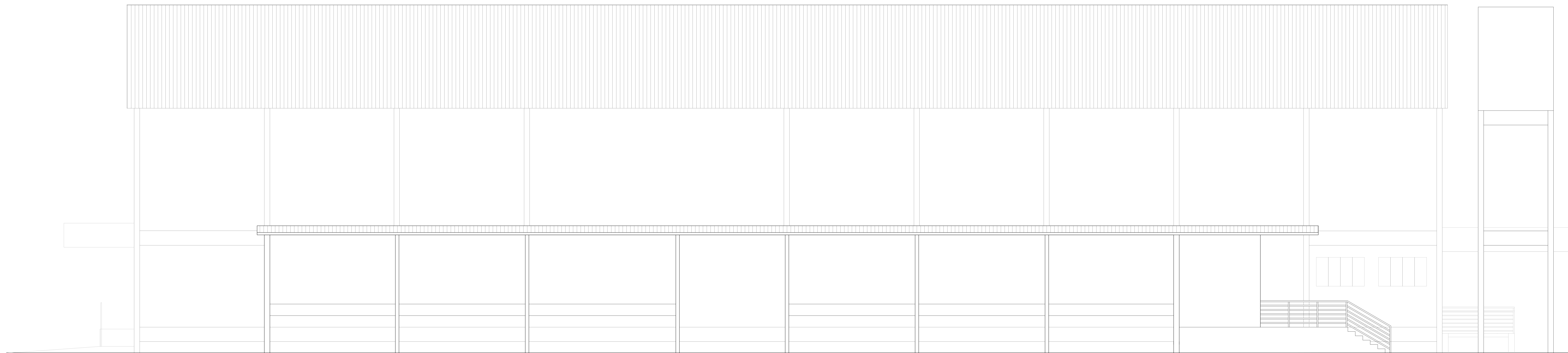
1 VISTA 03 ESCALA 1:50
