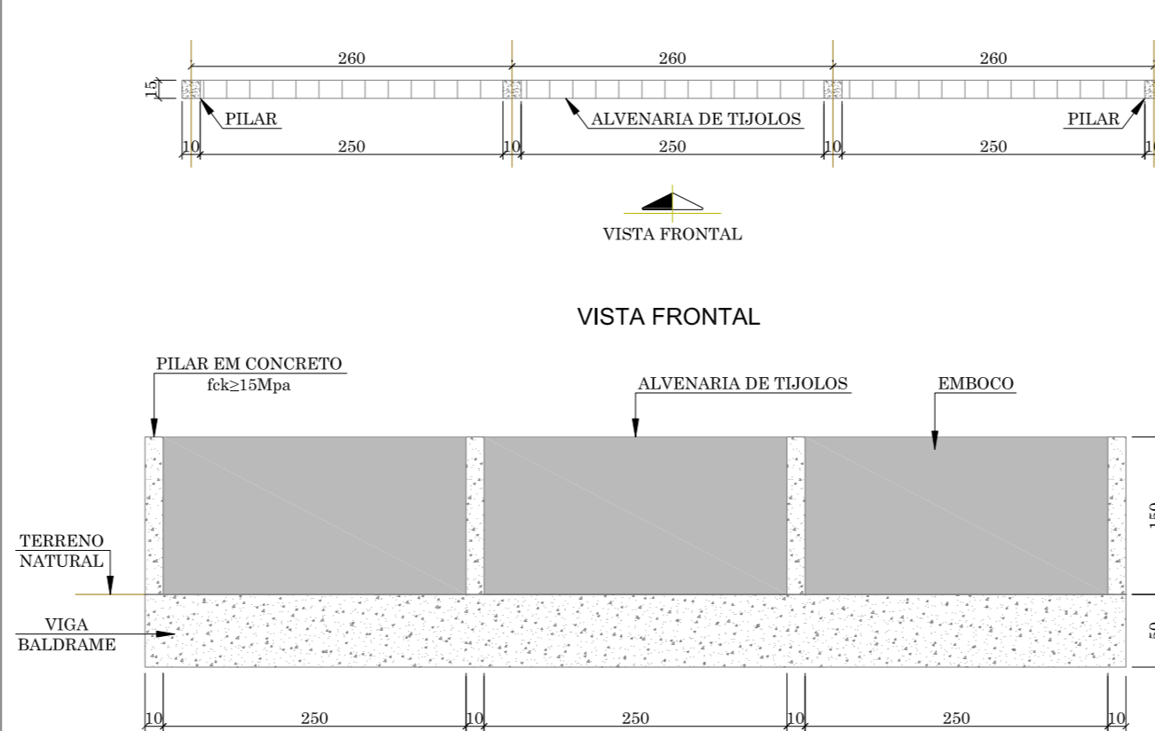
MURO DE ALVENARIA PLANTA BAIXA
