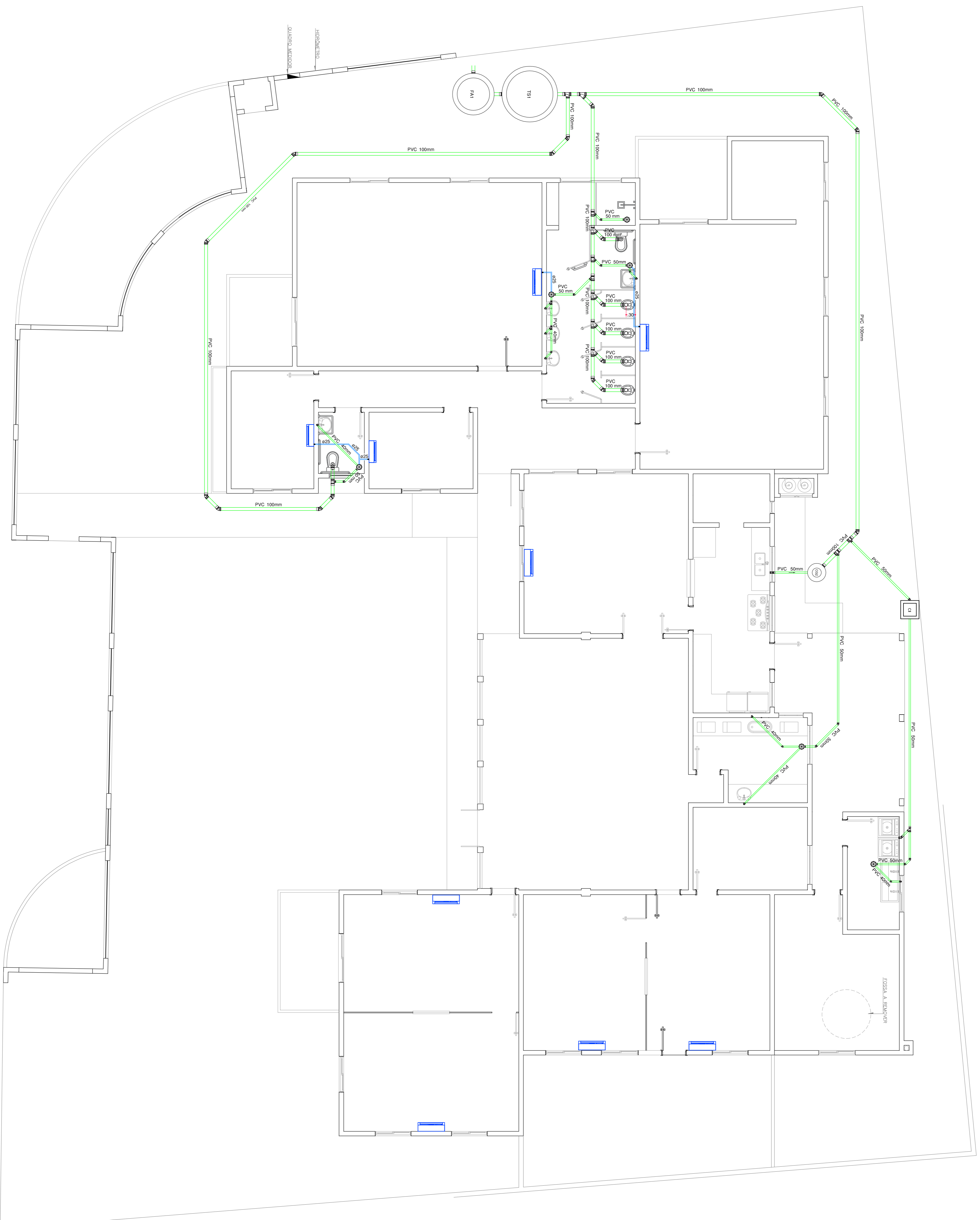
PLANTA DO SISTEMA DE ESGOTO – Superior – Esc. 1/50
