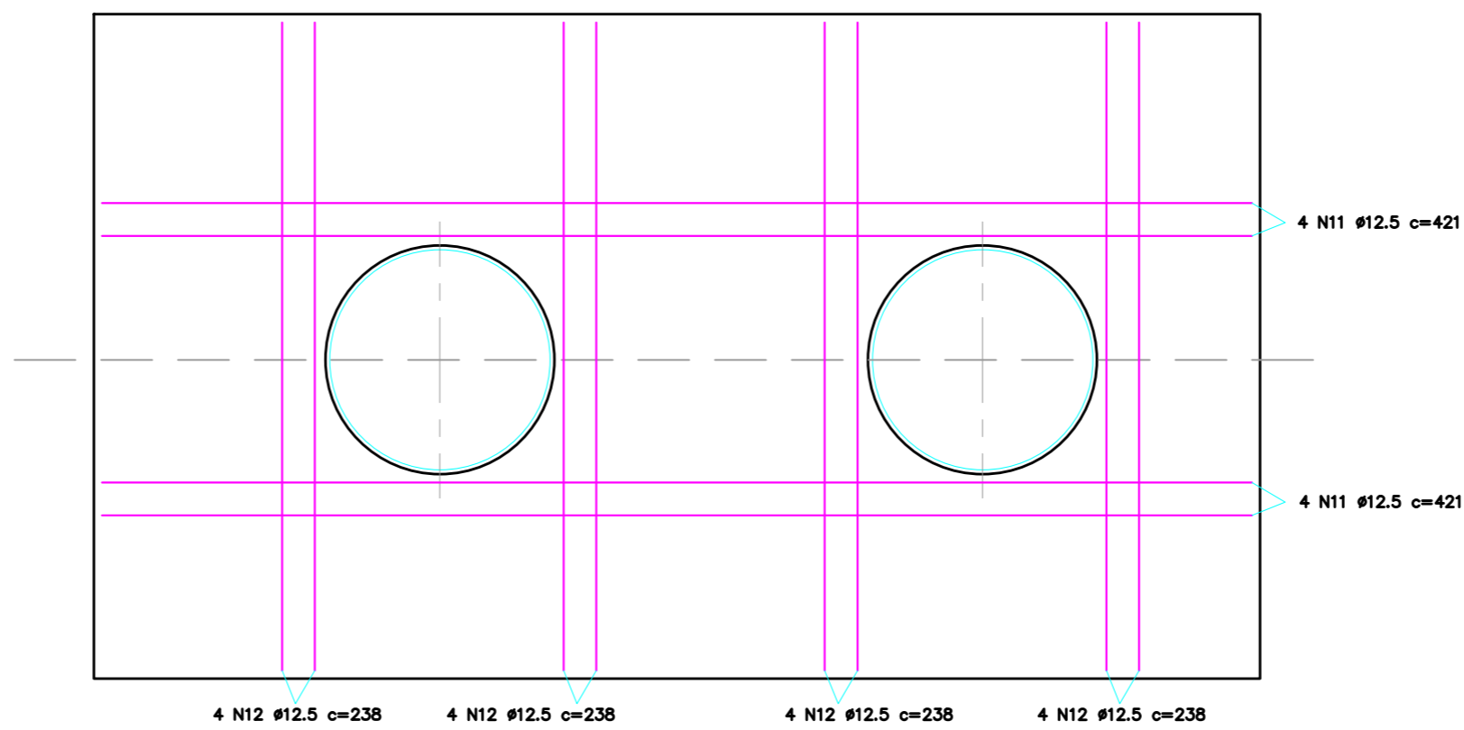
REFORÇO DE ABERTURAS ESC.: 1:25
