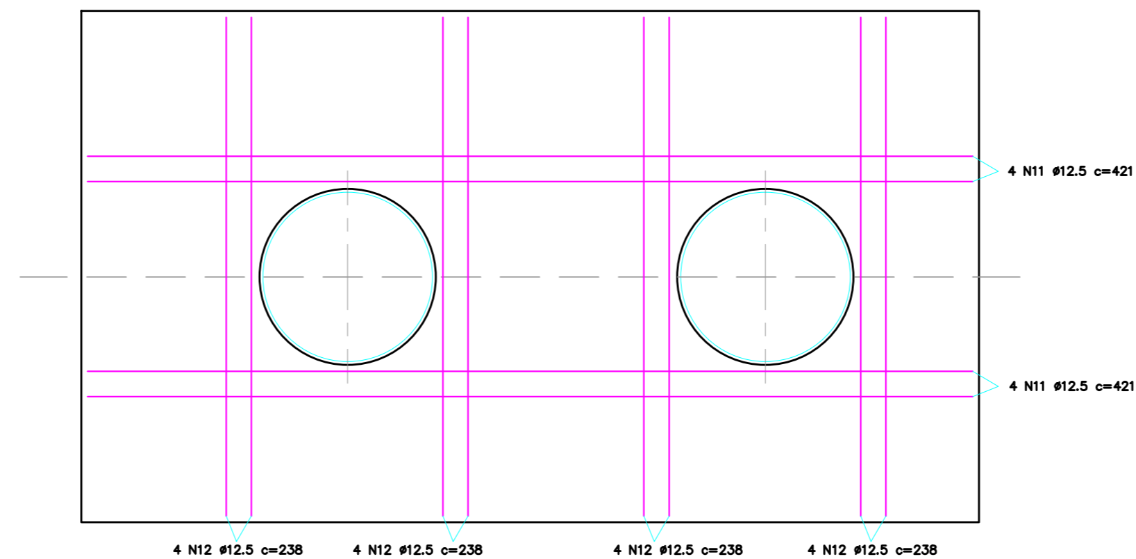
REFORÇO DE ABERTURAS ESC.: 1:25
